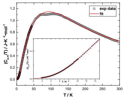
(b) C_{p,m}/T
