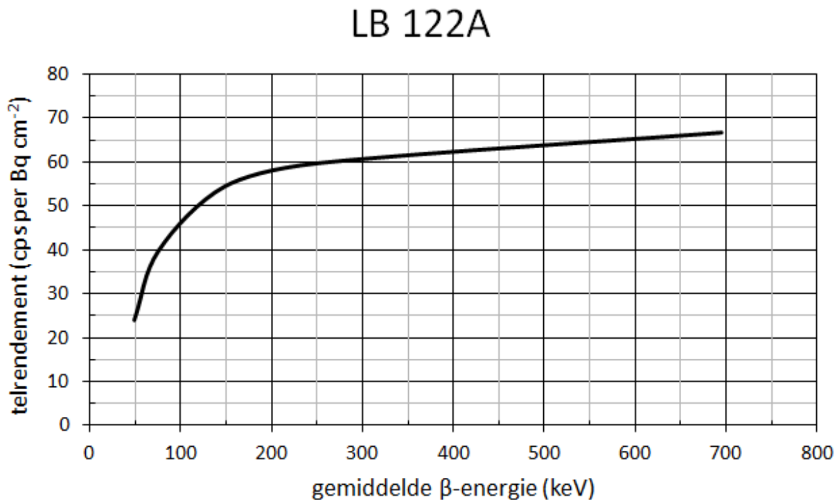
Figuur 4.1. Telrendement (in cps per Bq cm -2 ) van de besmettingsmonitor (Berthold LB 122A) als functie van de gemiddelde \beta -energie (in keV), uitgaande van een yield van 1.
